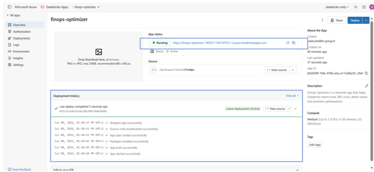
FIGURE 13 – Déploiement terminé.
